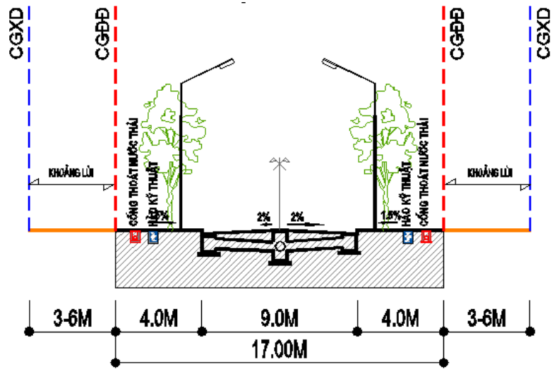
MẶT CẮT 2-2
